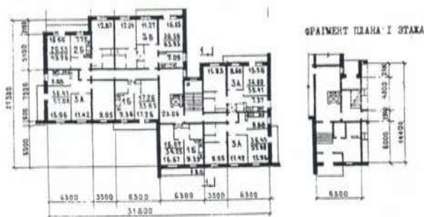
Экспликация квартир
